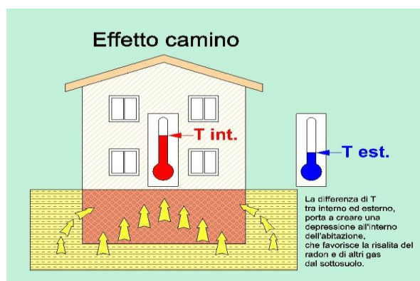
Figura 3: effetto camino
